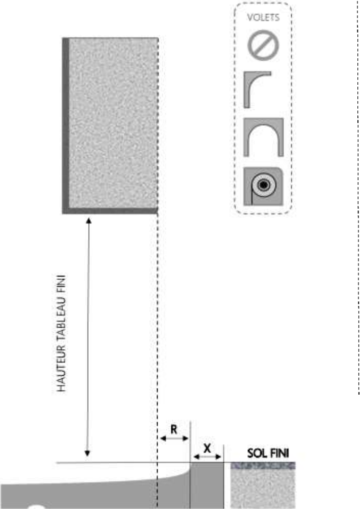
COUPE VERTICALE
