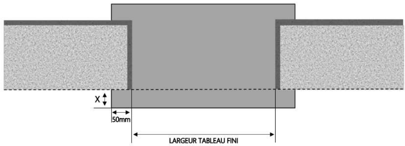
COUPE HORIZONTALE
