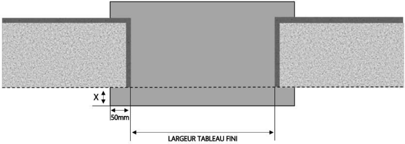
COUPE HORIZONTALE
