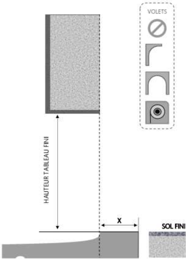
COUPE VERTICALE
