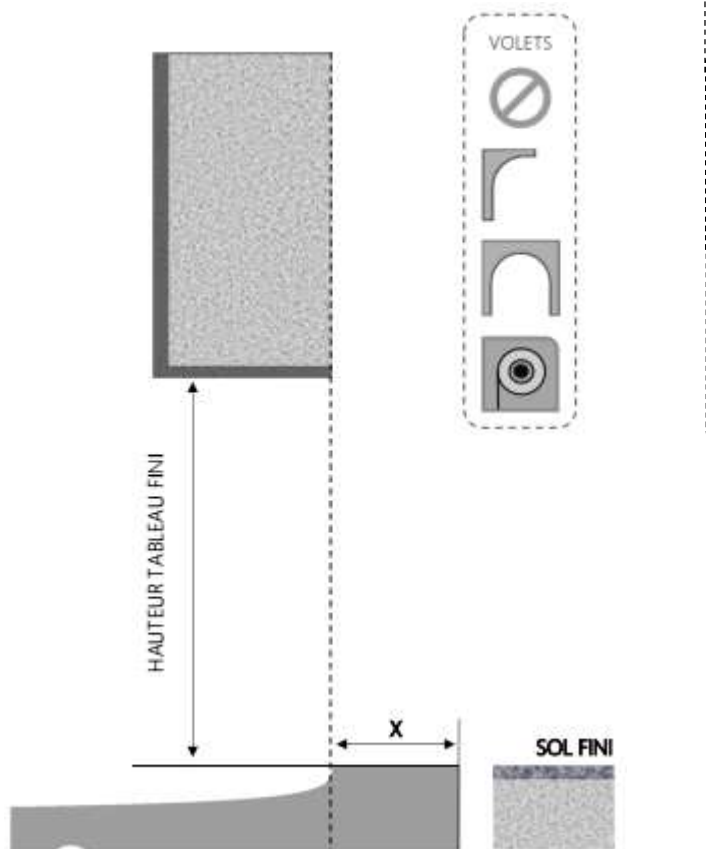
COUPE VERTICALE
