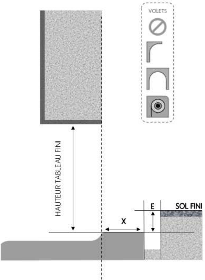
COUPE VERTICALE
