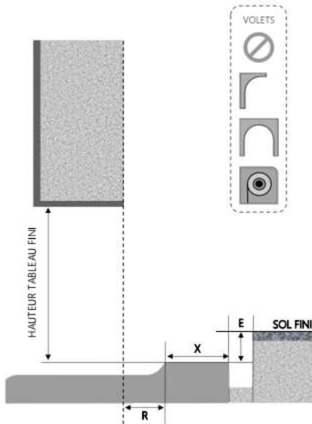
COUPE VERTICALE
