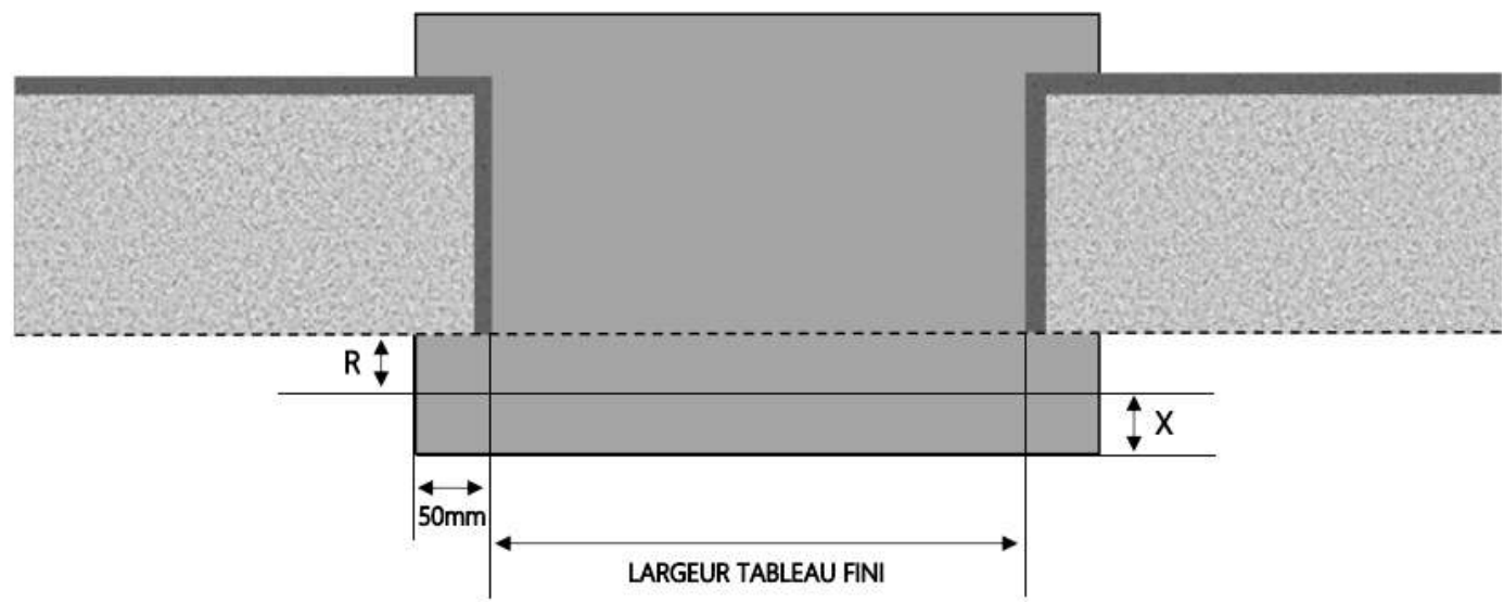
COUPE HORIZONTALE
