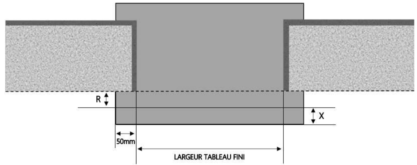
COUPE HORIZONTALE
