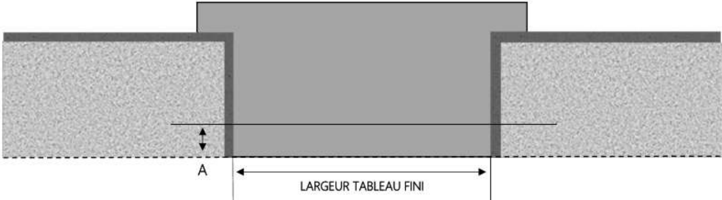
COUPE HORIZONTALE
