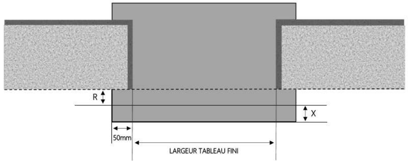
COUPE HORIZONTALE
