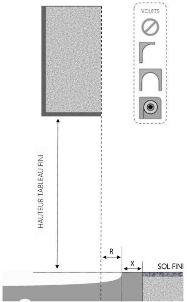
COUPE VERTICALE
