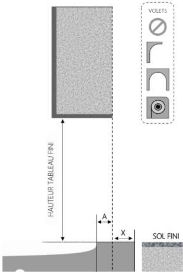
COUPE VERTICALE
