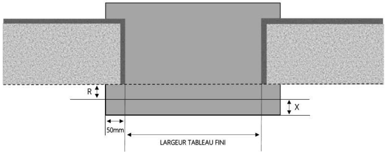
COUPE HORIZONTALE
