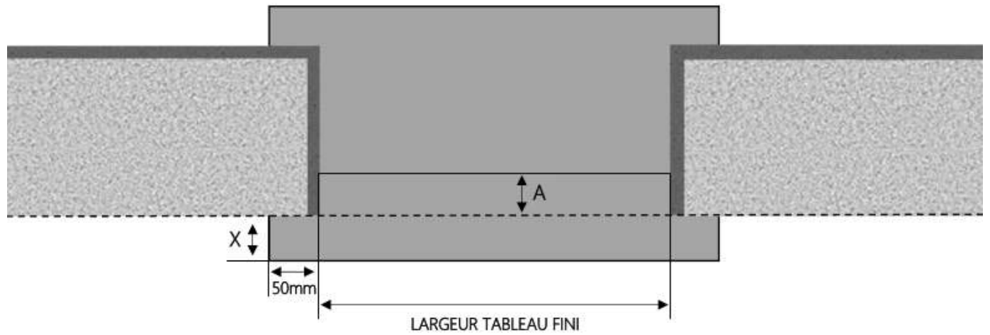
COUPE HORIZONTALE
