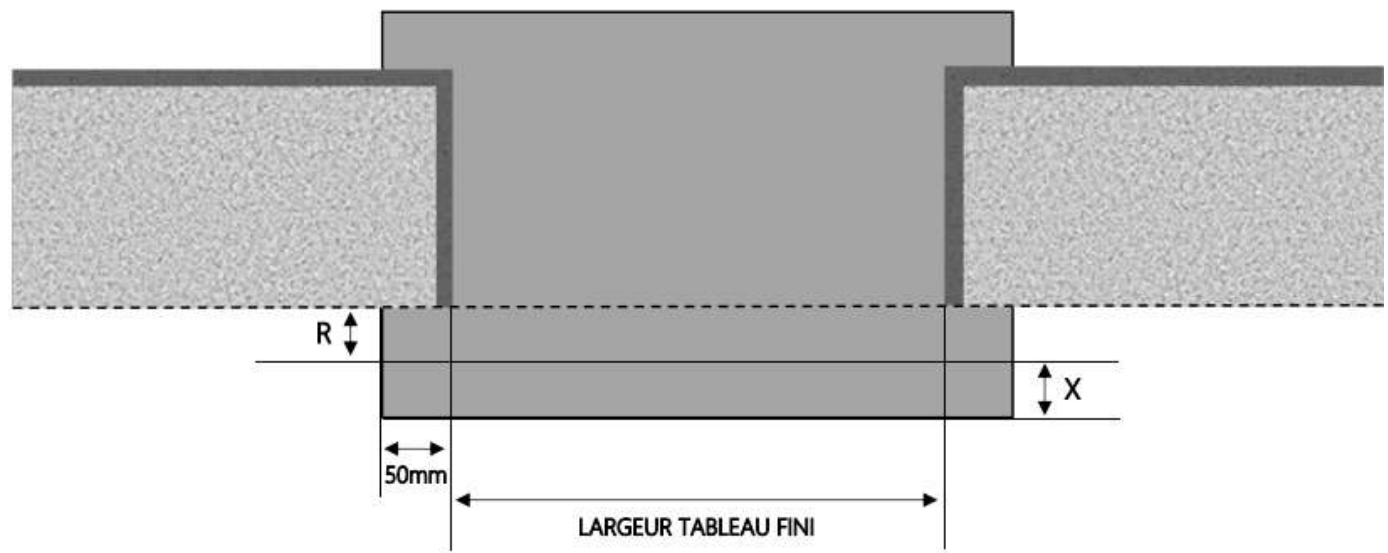
COUPE HORIZONTALE
