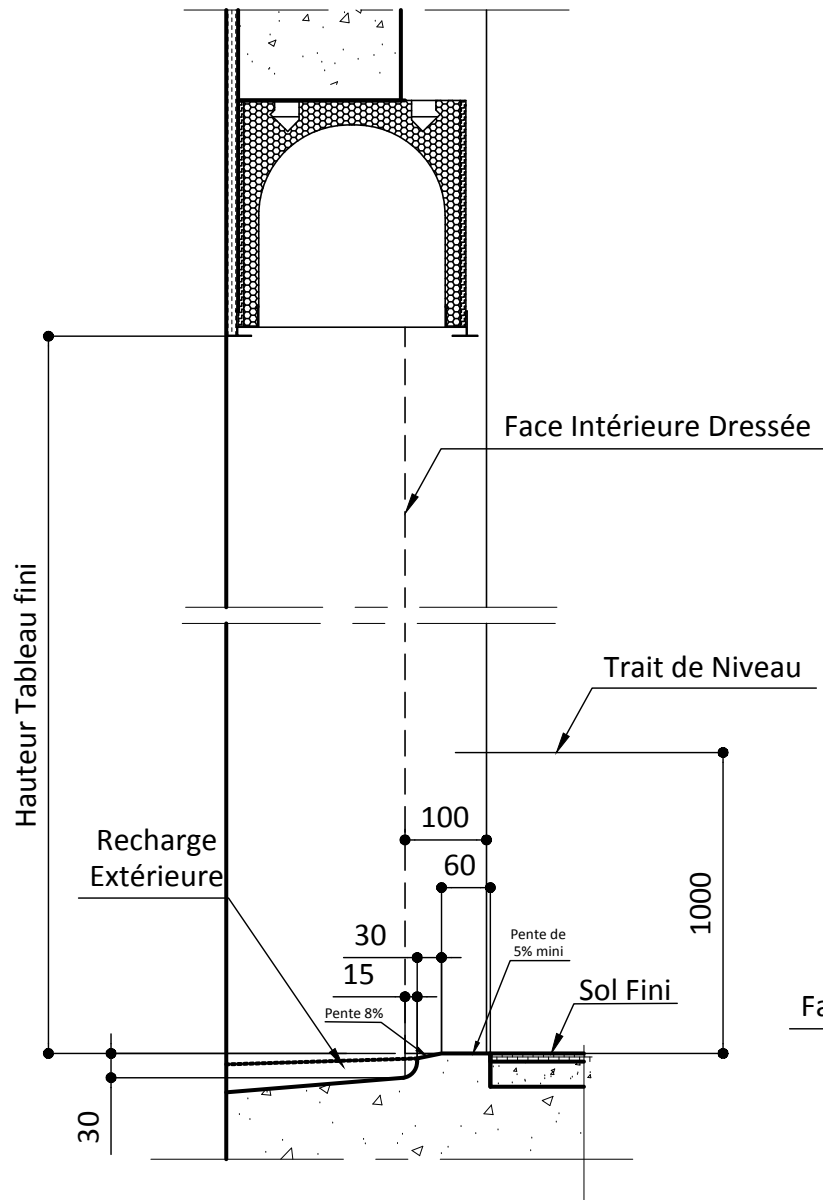
SEUIL PMR
