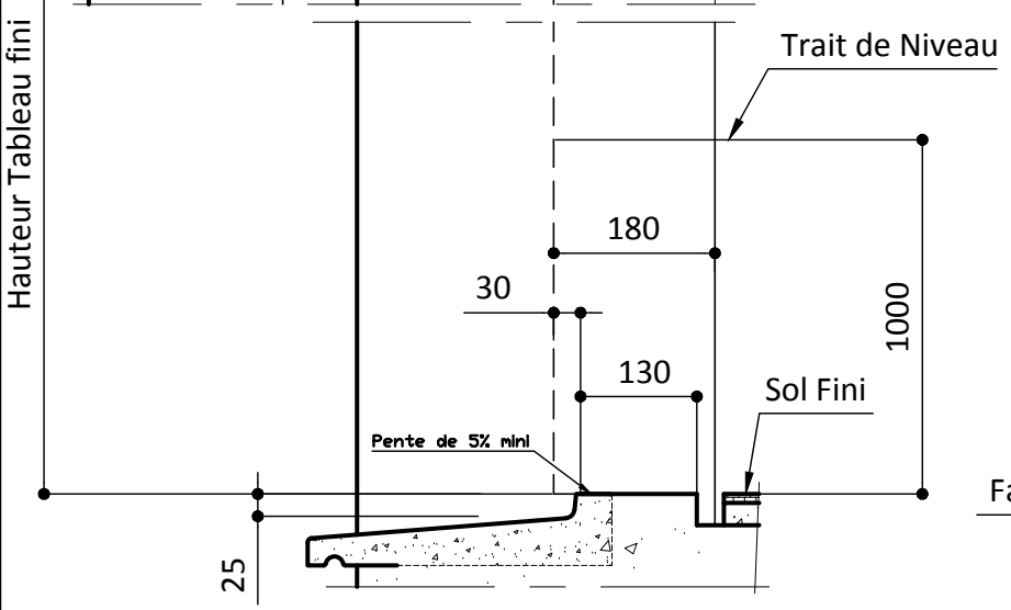
SEUIL STANDARD
