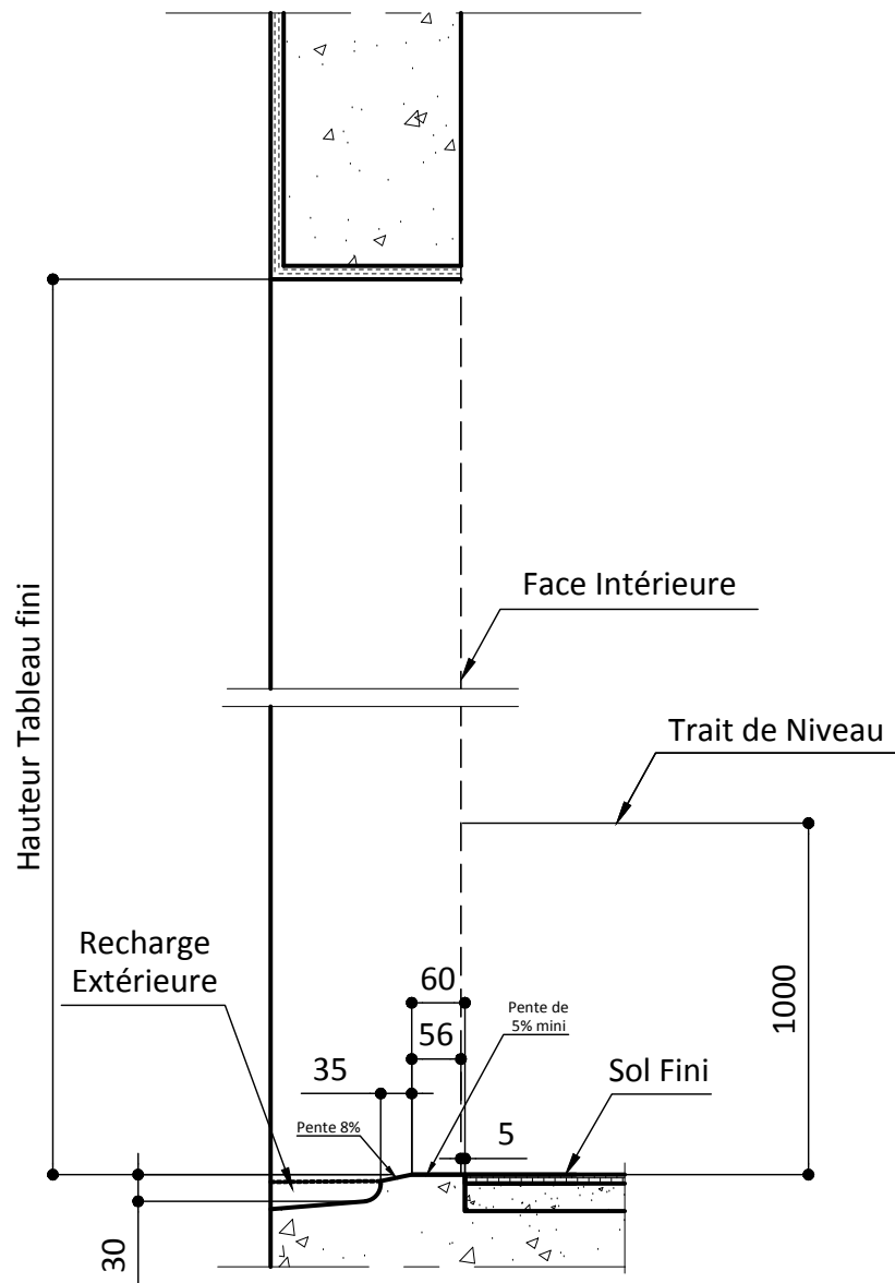
SEUIL PMR
