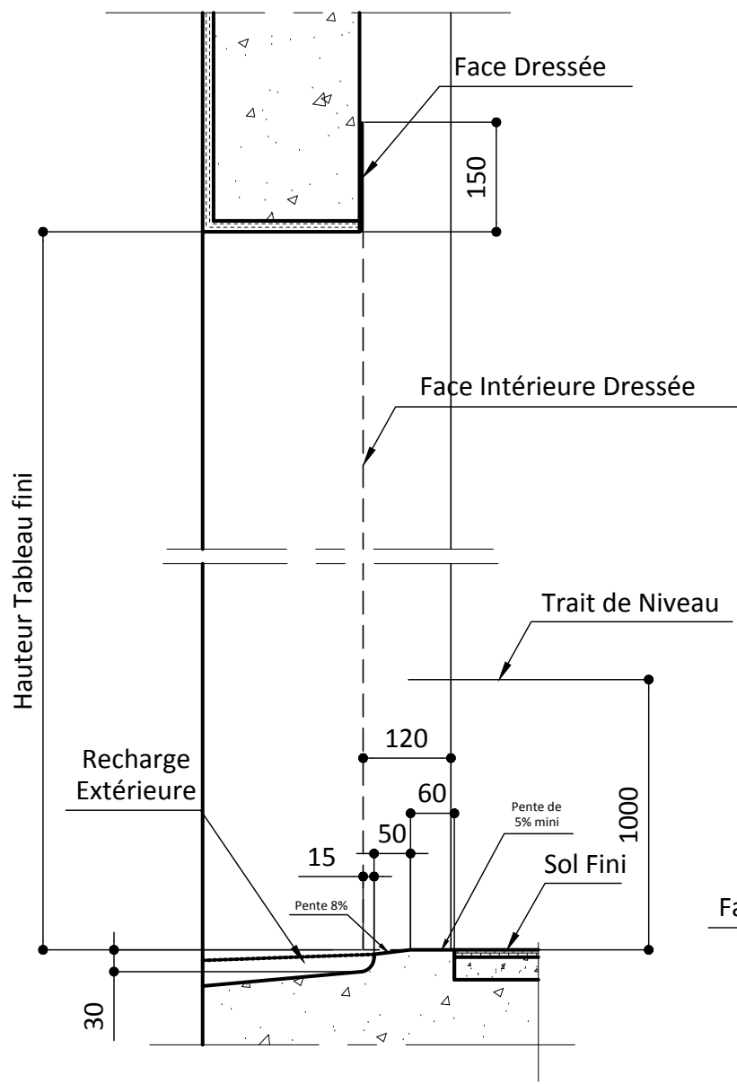
SEUIL PMR
