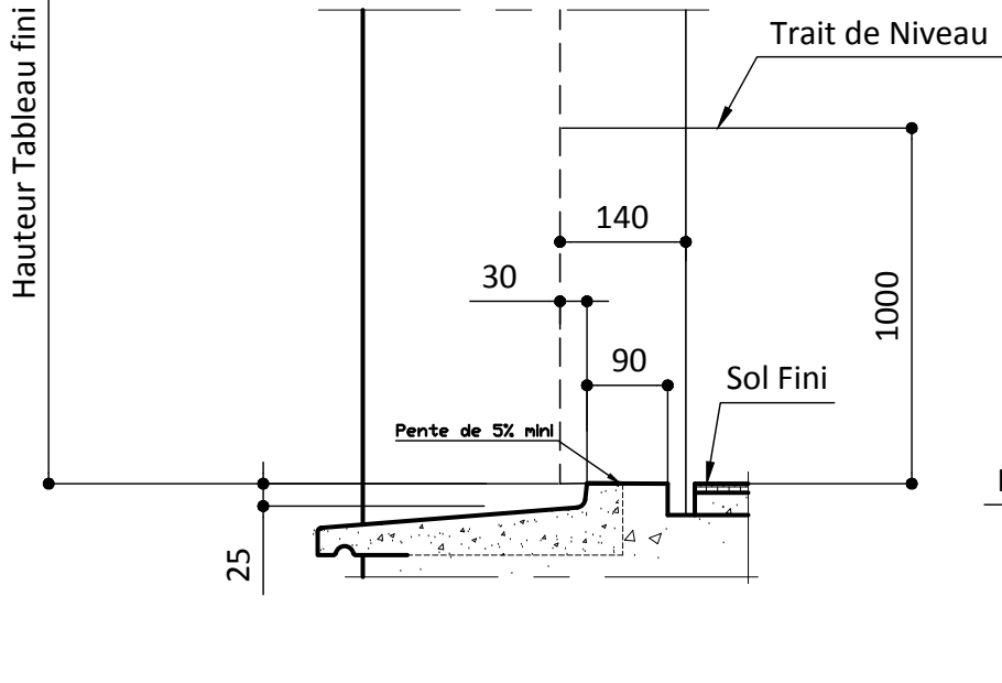
SEUIL STANDARD
