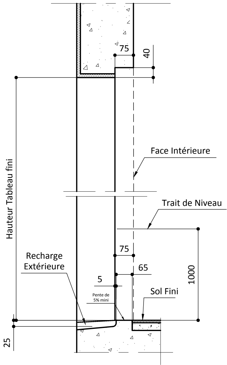
SEUIL PMR
