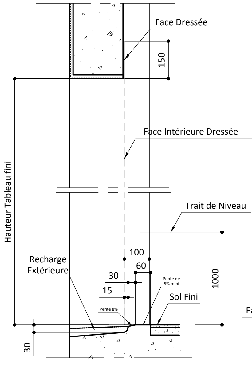
SEUIL PMR
