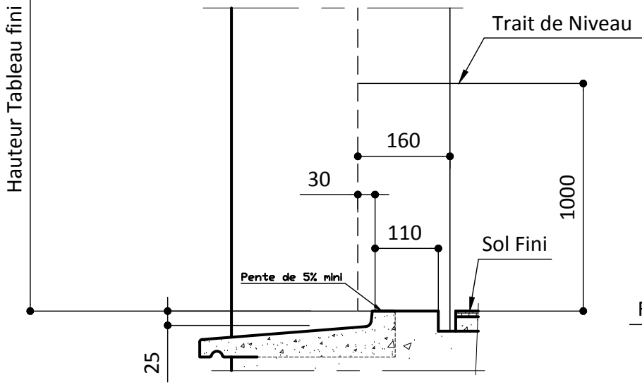
SEUIL STANDARD
