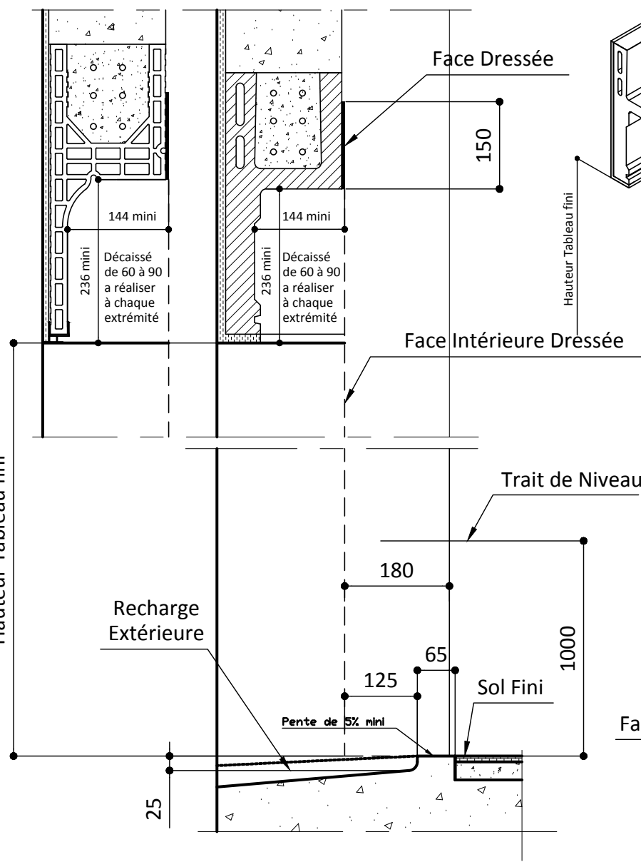
SEUIL PMR
