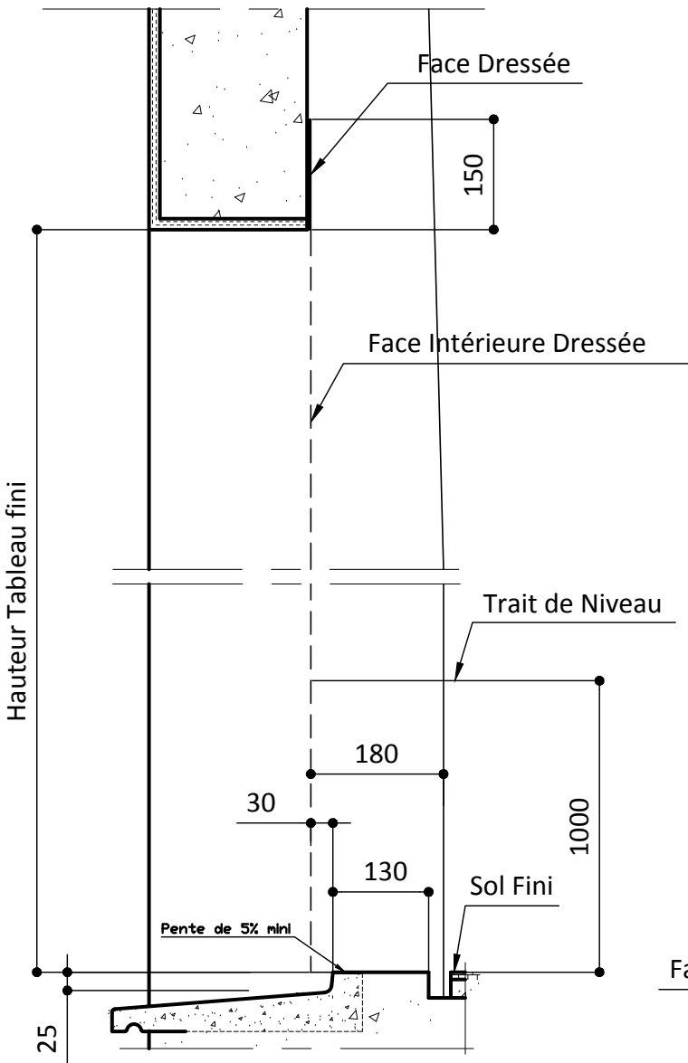
SEUIL STANDARD
