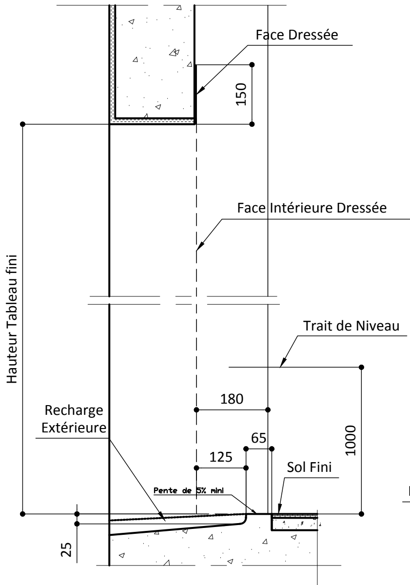
SEUIL PMR
