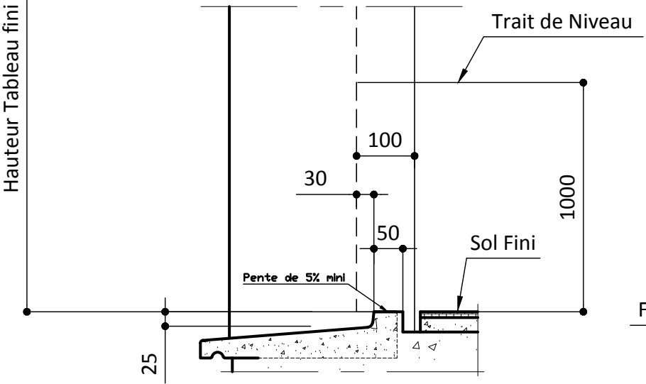
SEUIL STANDARD
