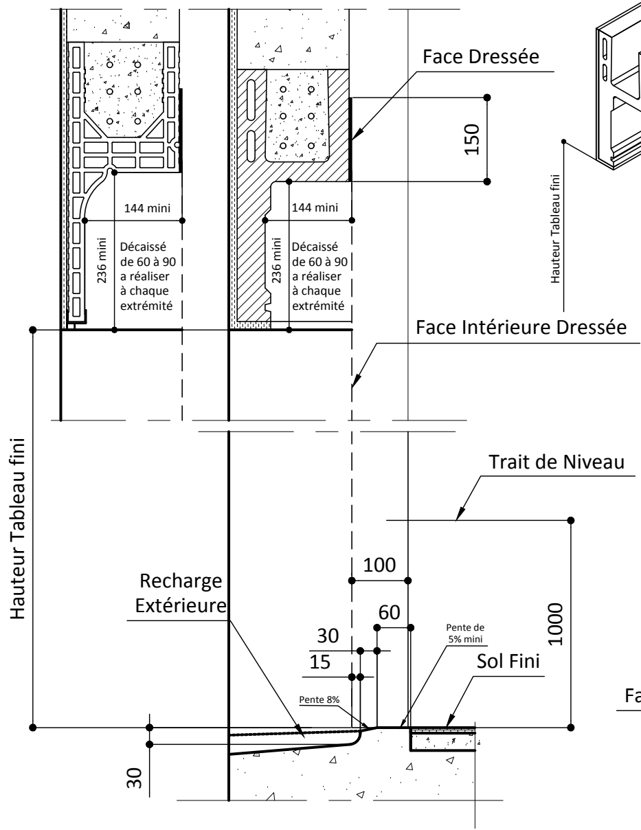
SEUIL PMR
