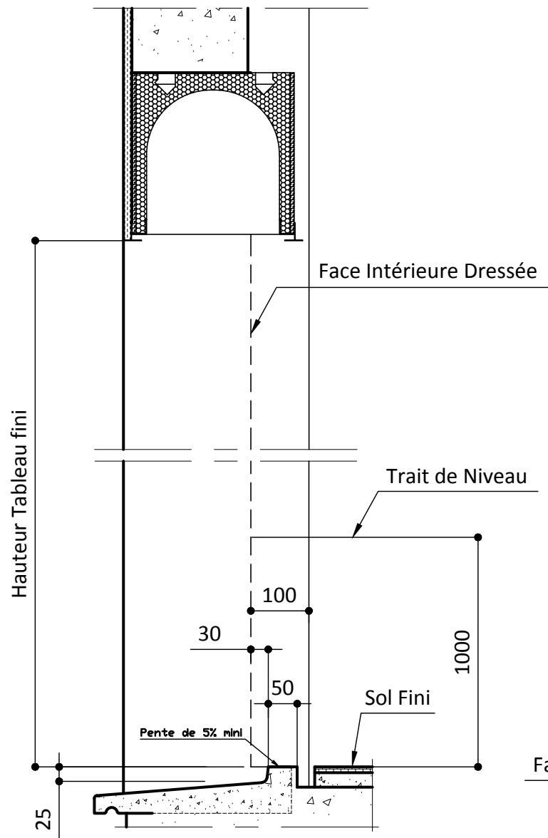
SEUIL STANDARD
