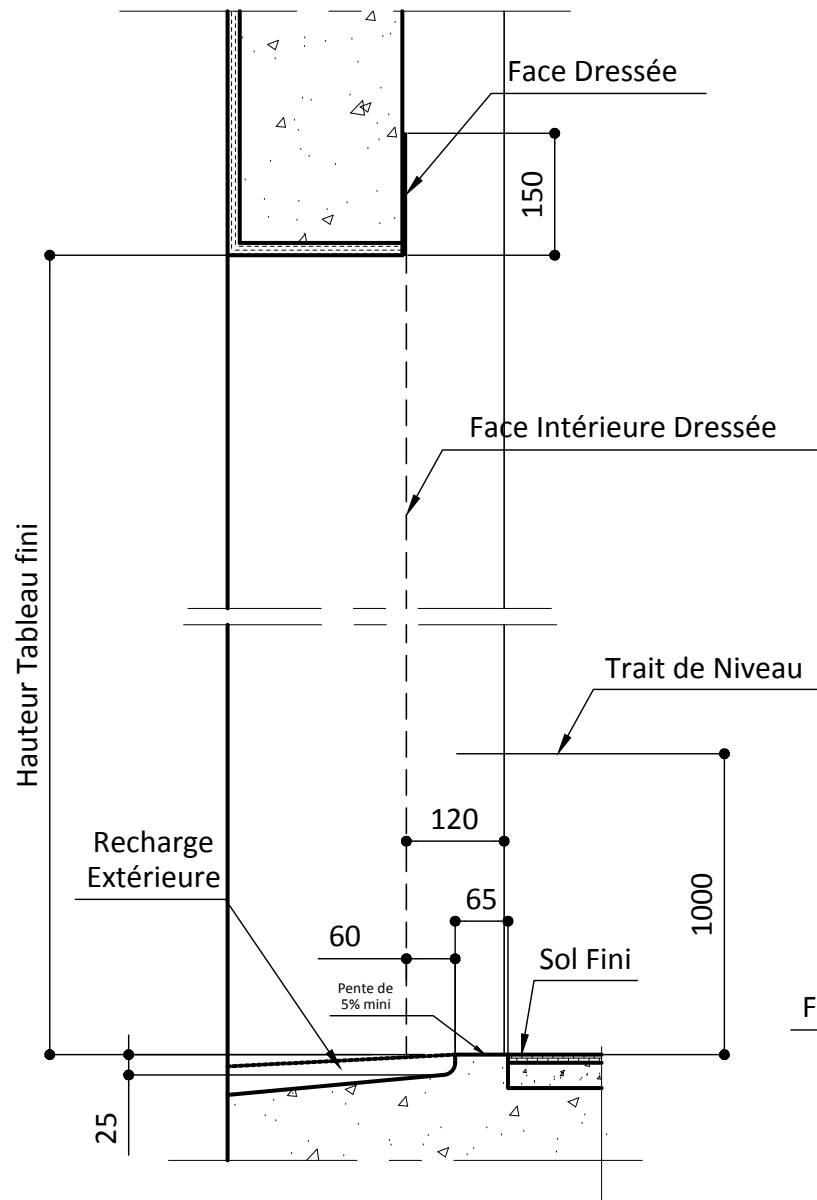
SEUIL PMR
