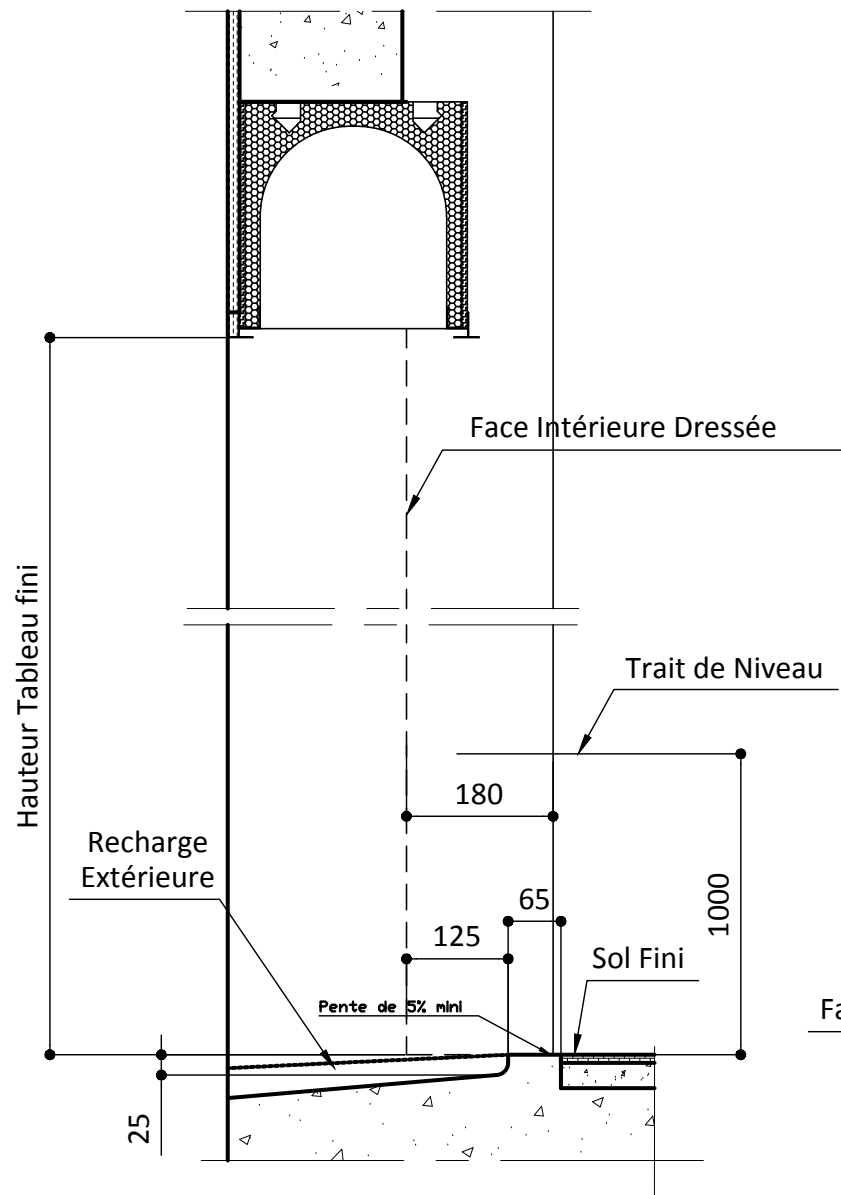
SEUIL PMR
