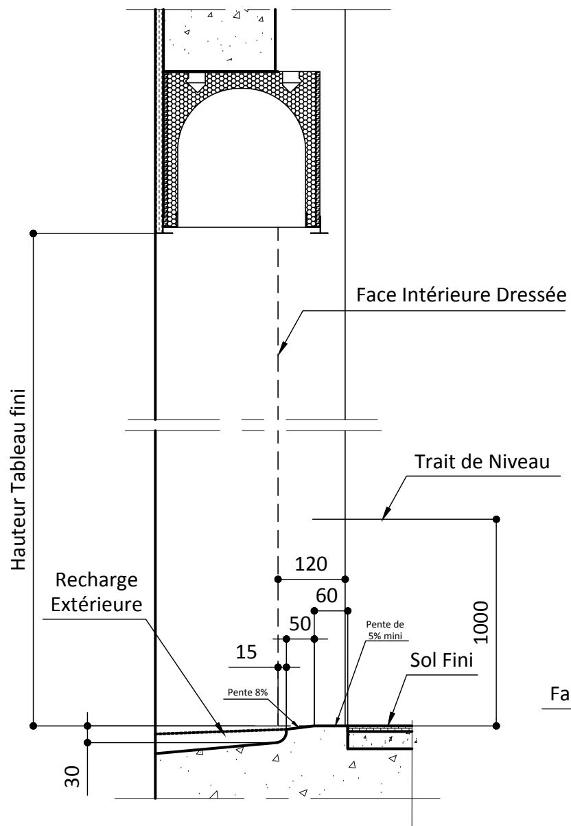
SEUIL PMR
