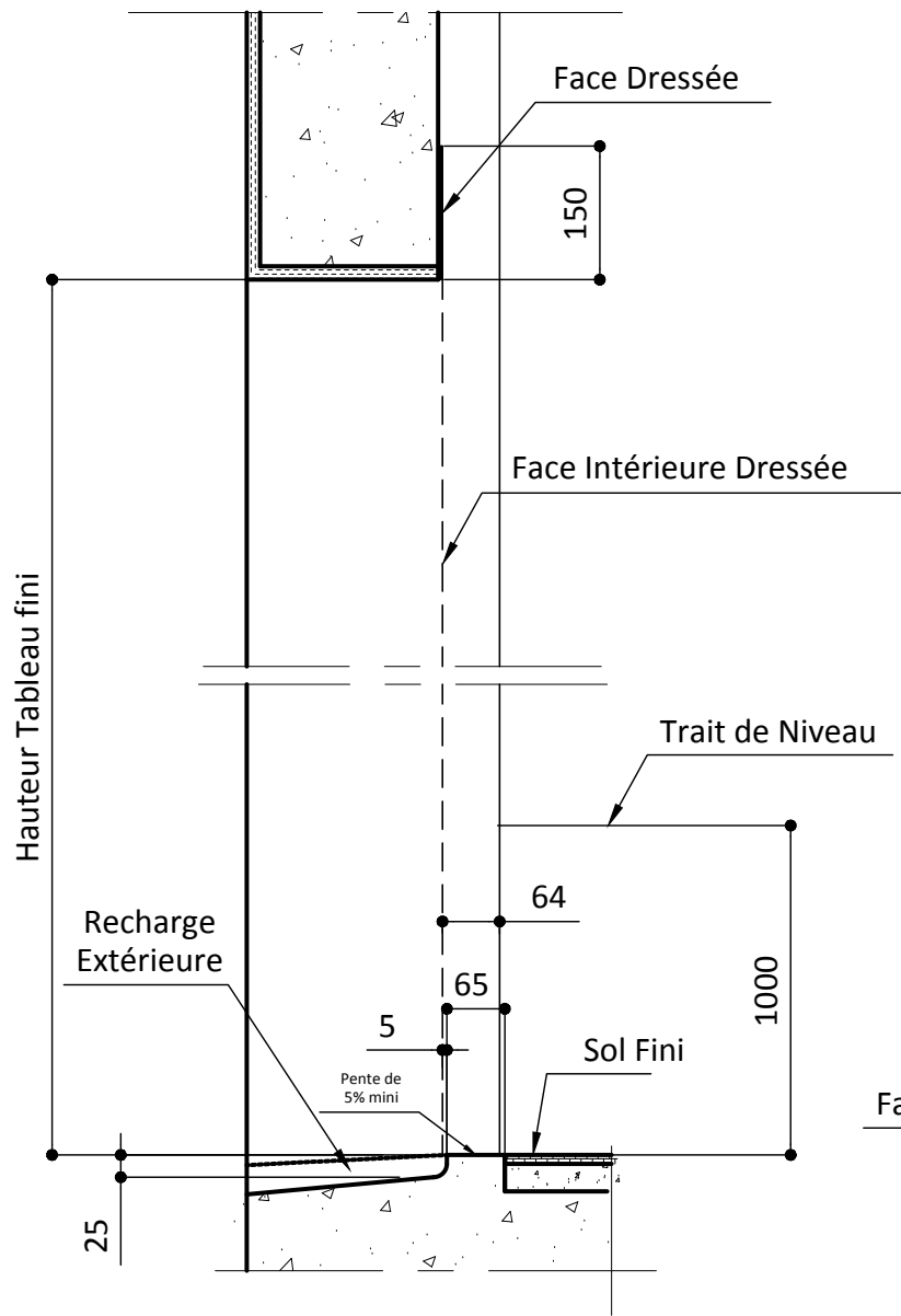
SEUIL PMR
