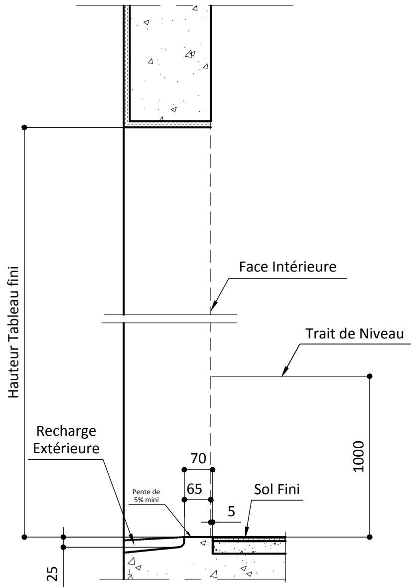
SEUIL PMR
