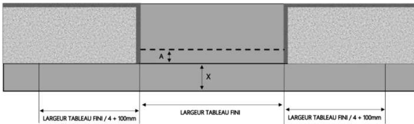
COUPE HORIZONTALE
