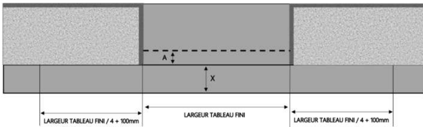
COUPE HORIZONTALE
