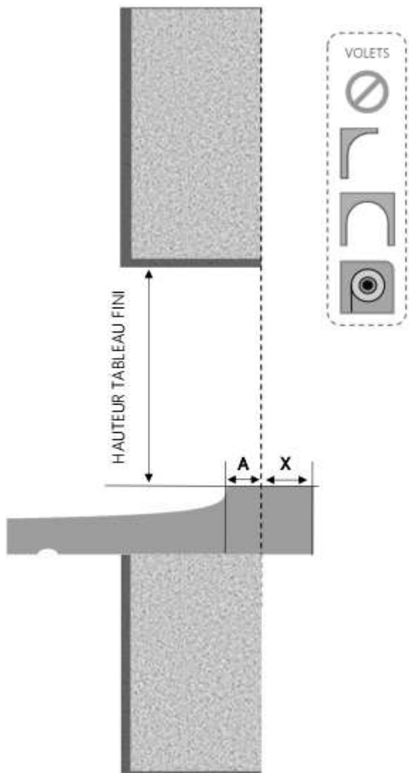
COUPE VERTICALE
