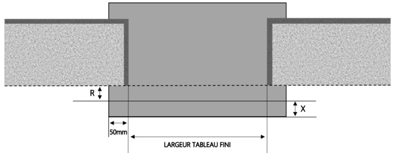
COUPE HORIZONTALE
