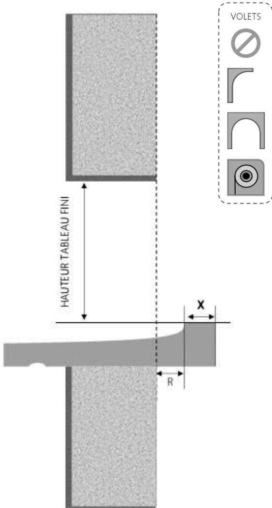
COUPE VERTICALE
