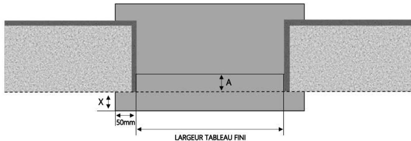
COUPE HORIZONTALE
