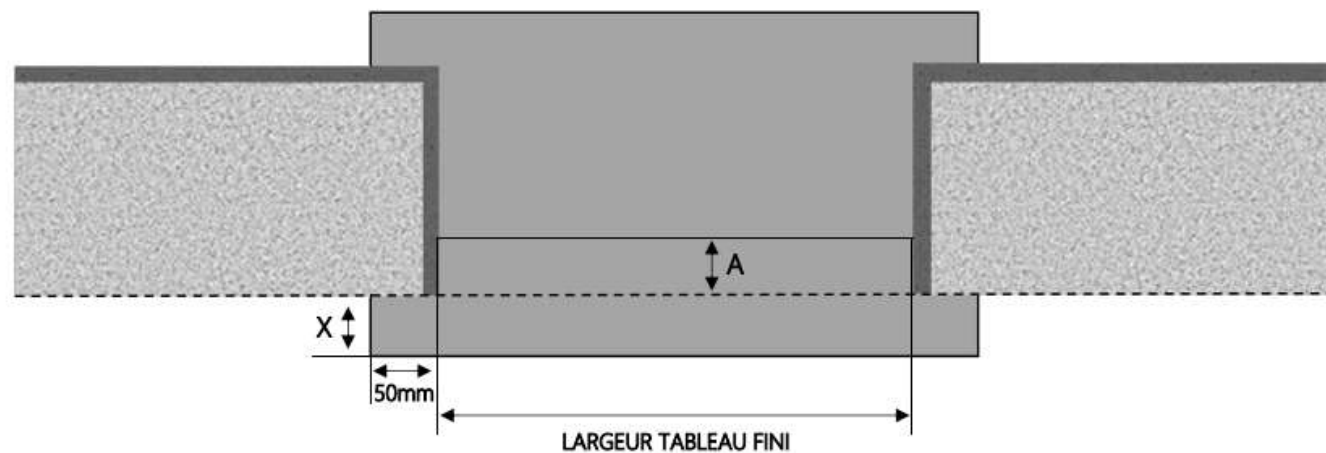
COUPE HORIZONTALE
