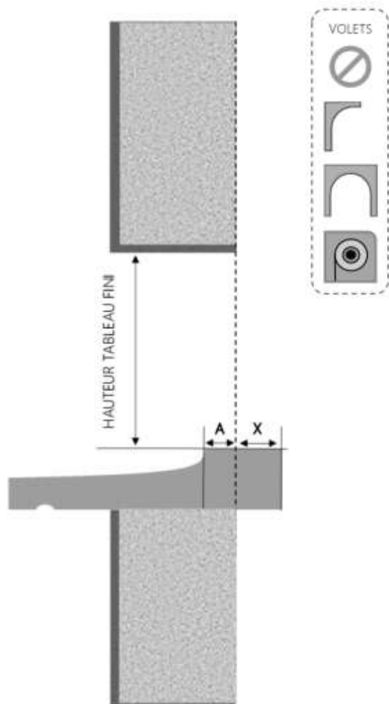
COUPE VERTICALE
