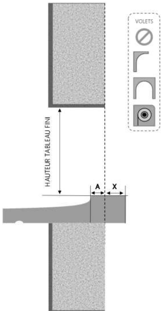
COUPE VERTICALE
