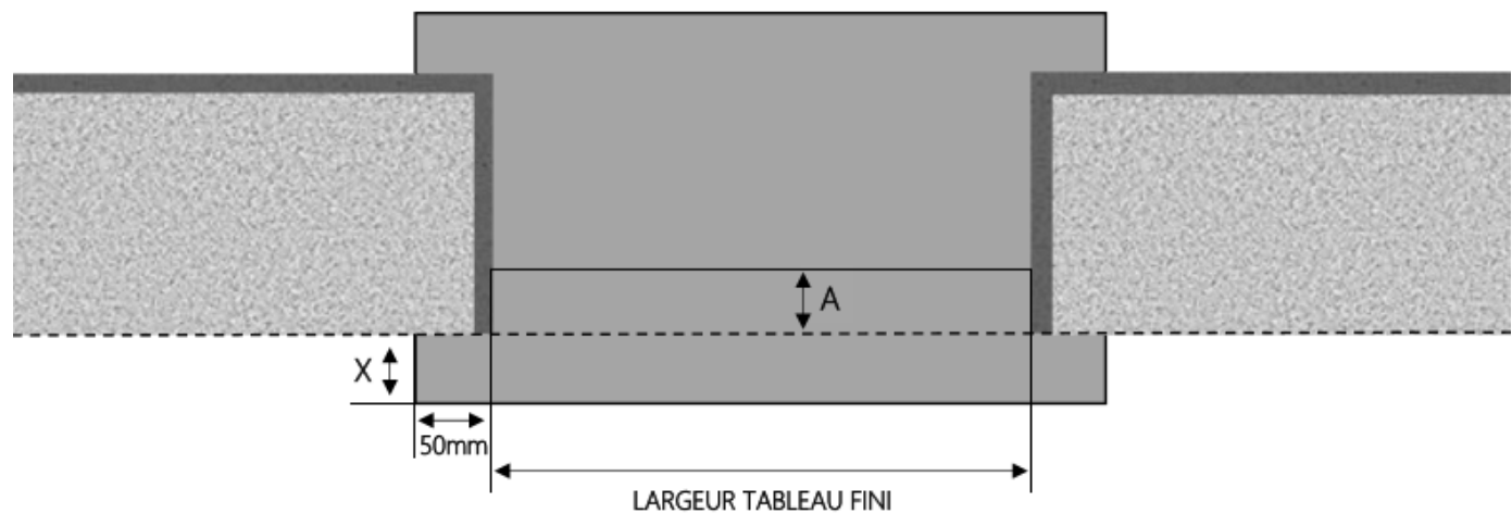
COUPE HORIZONTALE
