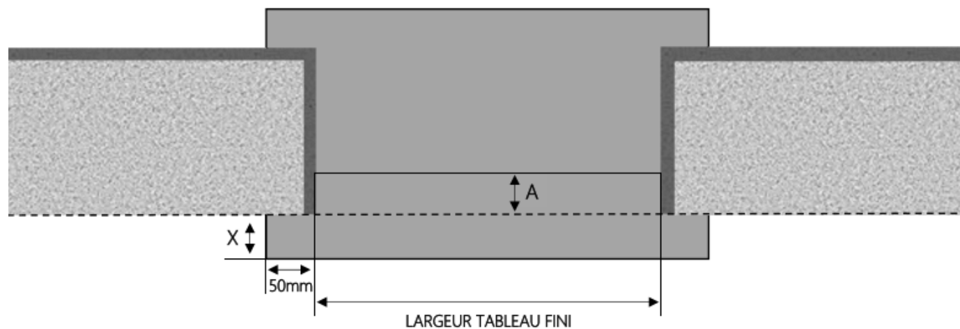
COUPE HORIZONTALE
