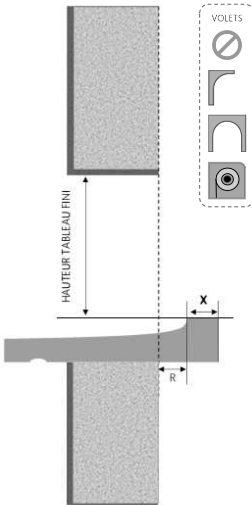
COUPE VERTICALE
