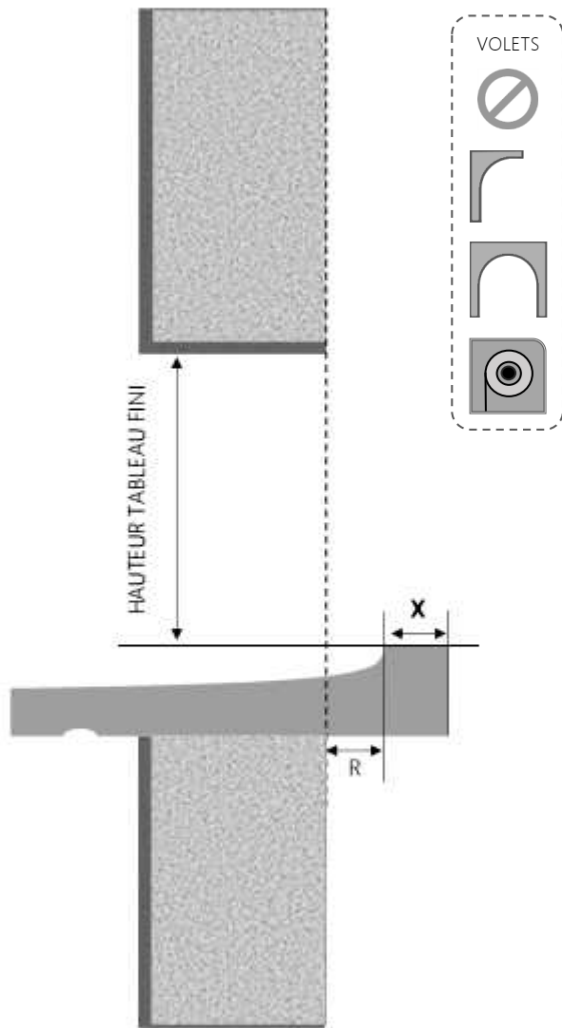
COUPE VERTICALE
