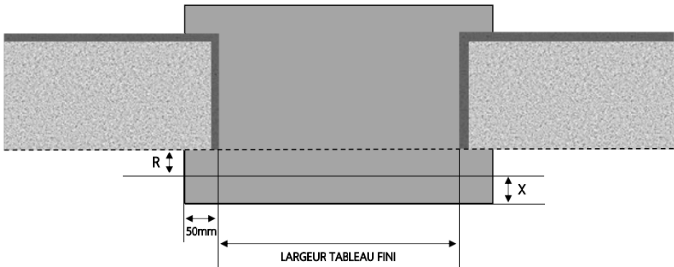
COUPE HORIZONTALE
