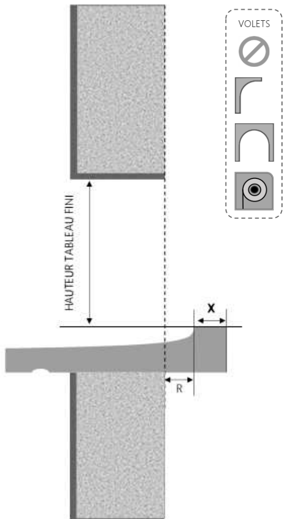
COUPE VERTICALE
