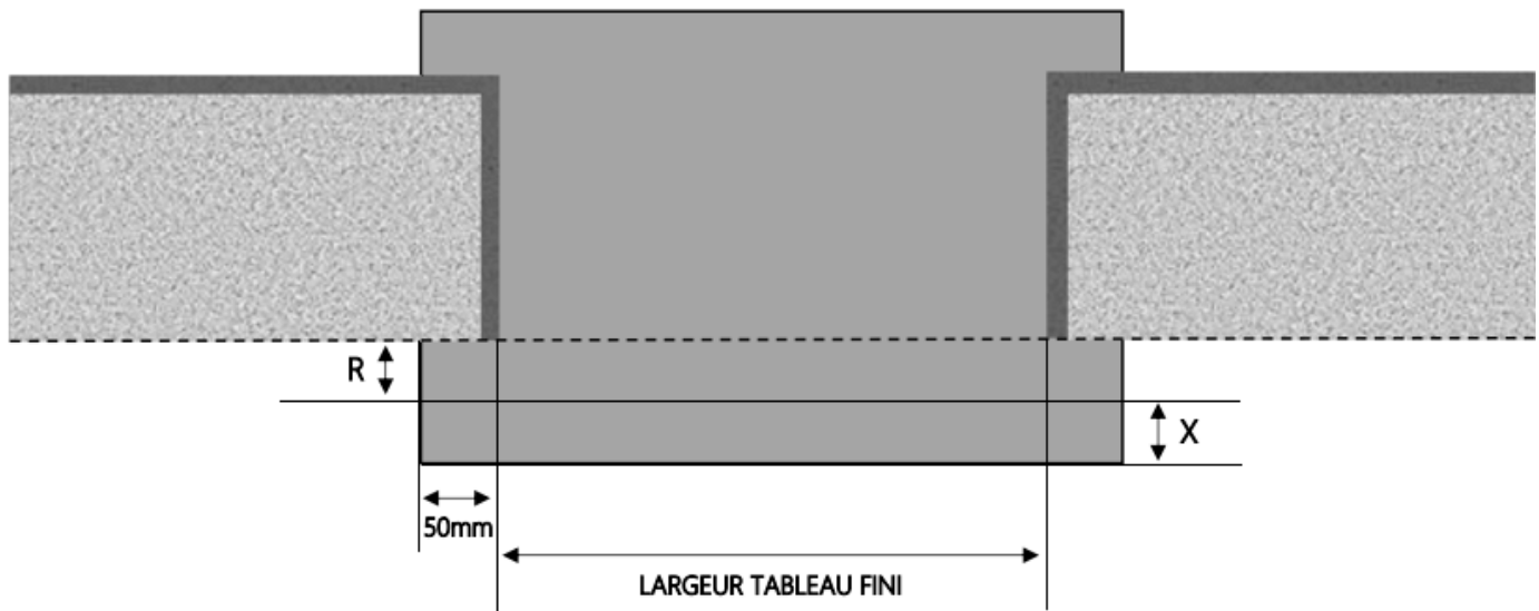
COUPE HORIZONTALE
