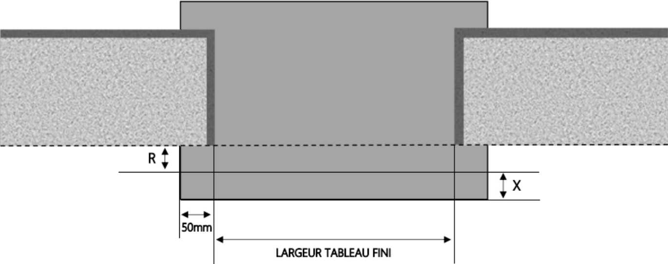
COUPE HORIZONTALE
