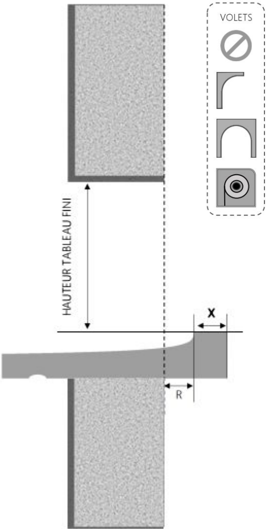
COUPE VERTICALE
