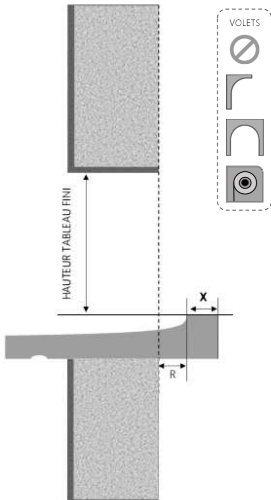
COUPE VERTICALE
