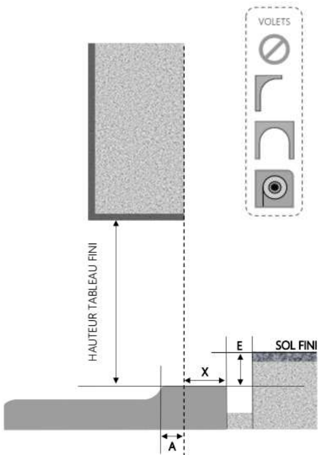
COUPE VERTICALE
