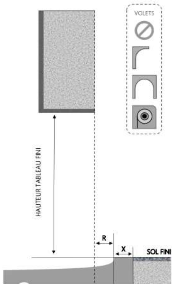
COUPE VERTICALE
