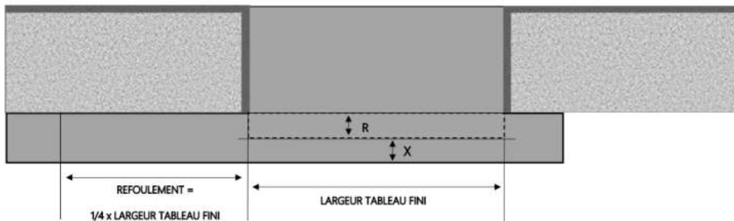
COUPE HORIZONTALE
