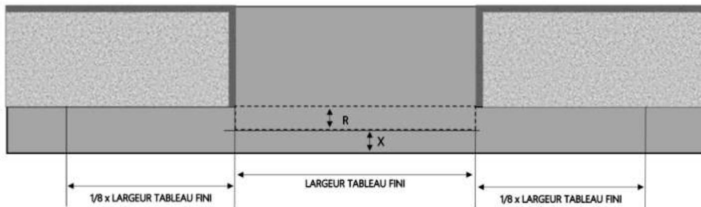
COUPE HORIZONTALE
