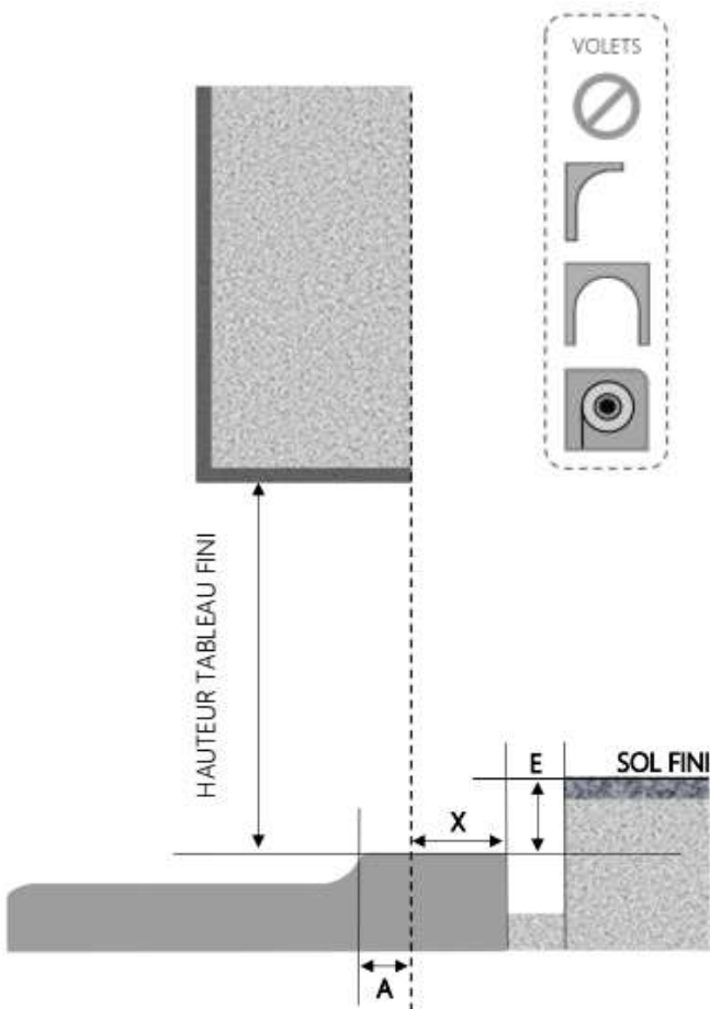
COUPE VERTICALE
