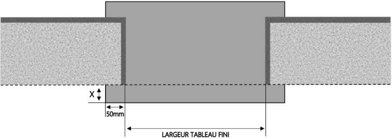
COUPE HORIZONTALE
