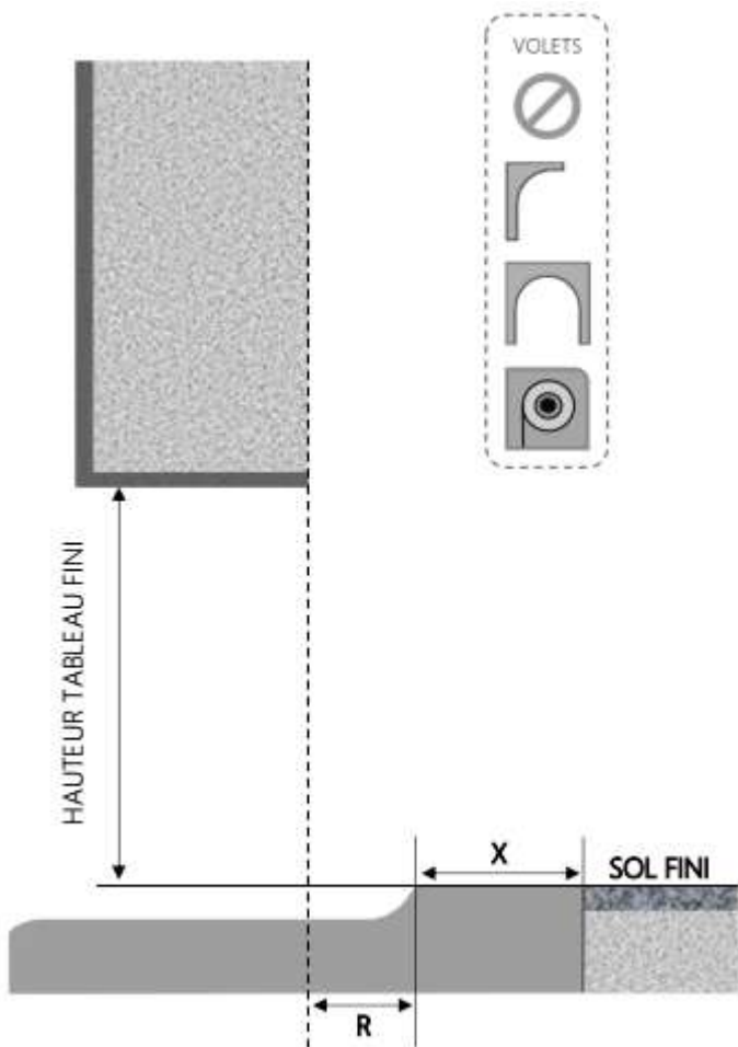
COUPE VERTICALE
