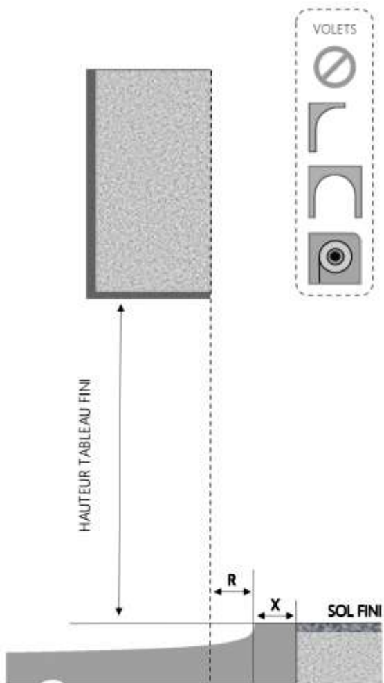
COUPE VERTICALE
