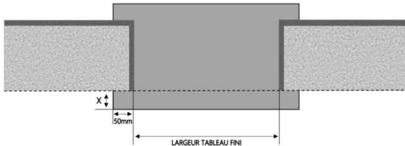
COUPE HORIZONTALE
