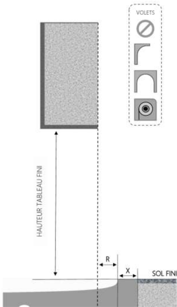
COUPE VERTICALE
