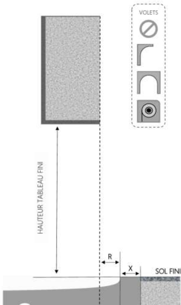
COUPE VERTICALE
