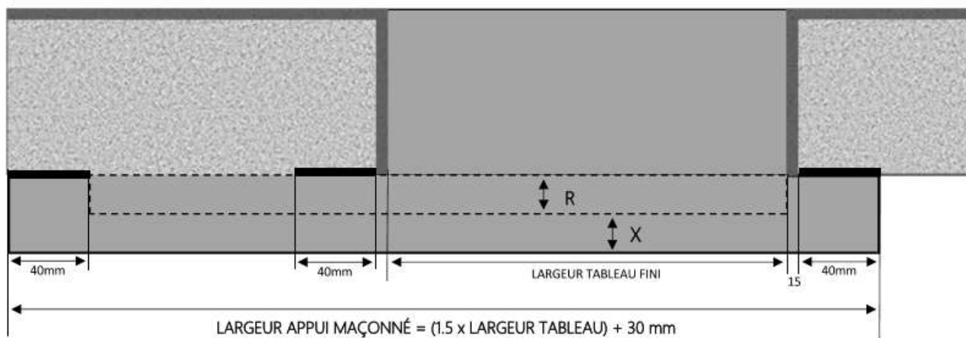
COUPE HORIZONTALE
