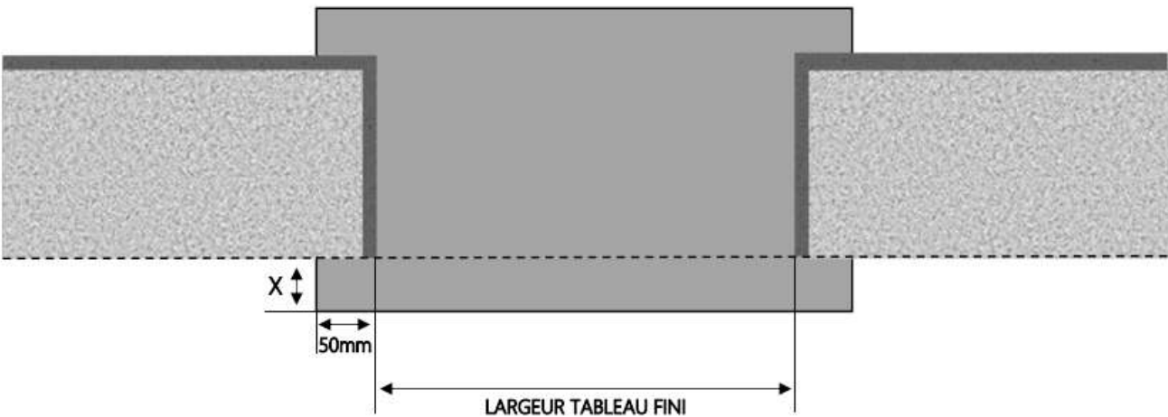
COUPE HORIZONTALE
