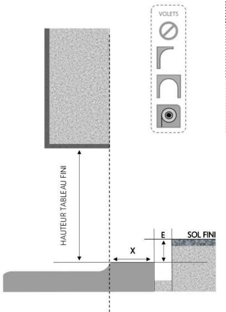
COUPE VERTICALE
