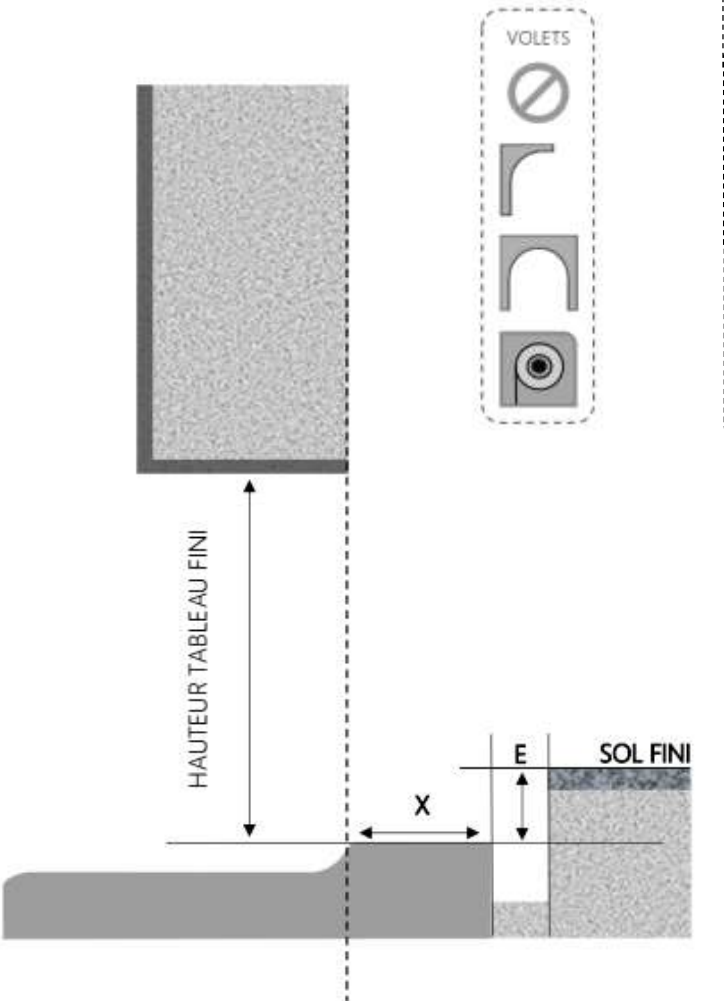
COUPE VERTICALE
