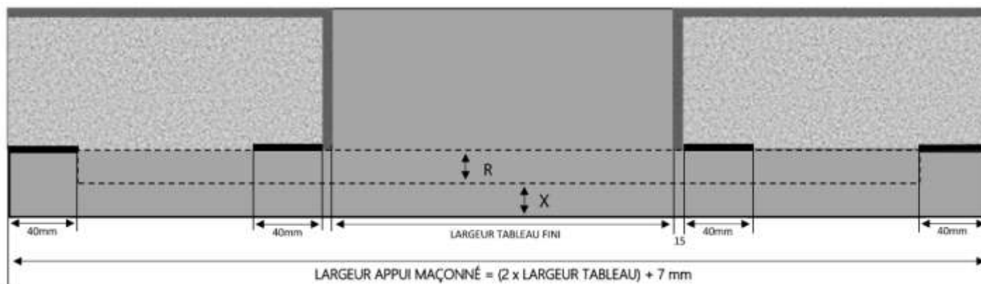
COUPE HORIZONTALE
