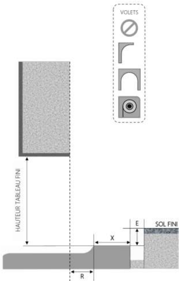
COUPE VERTICALE
