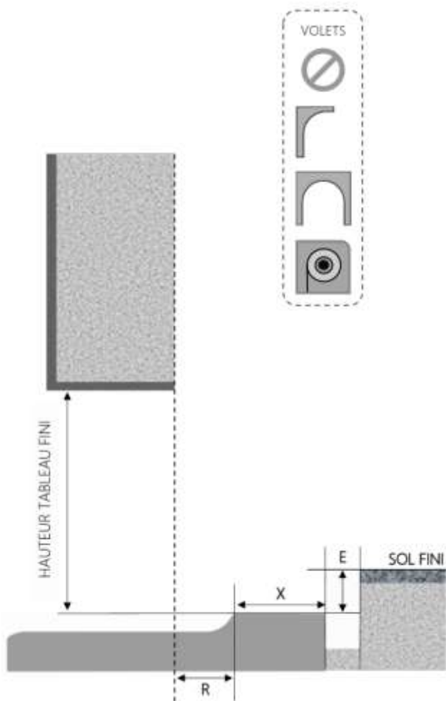
COUPE VERTICALE
