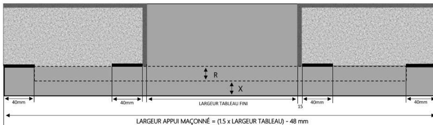
COUPE HORIZONTALE
