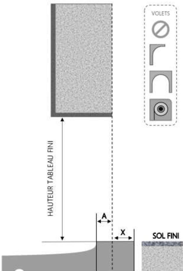
COUPE VERTICALE
