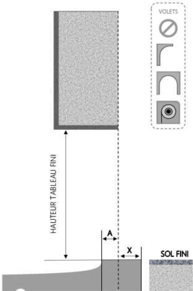
COUPE VERTICALE
