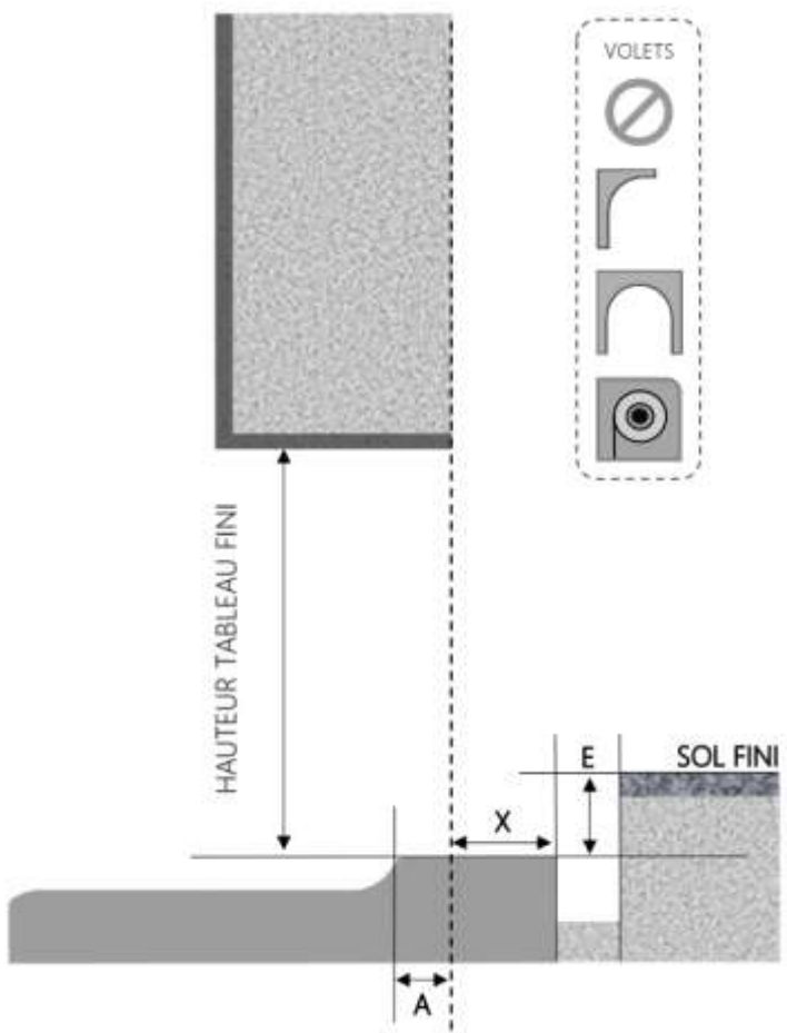
COUPE VERTICALE
