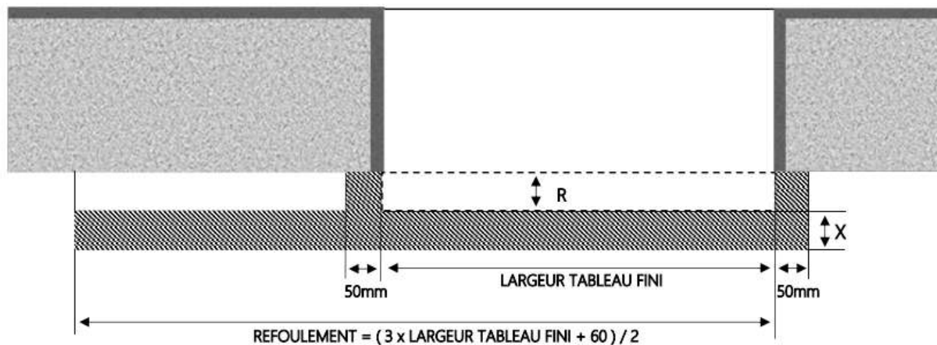
COUPE HORIZONTALE
