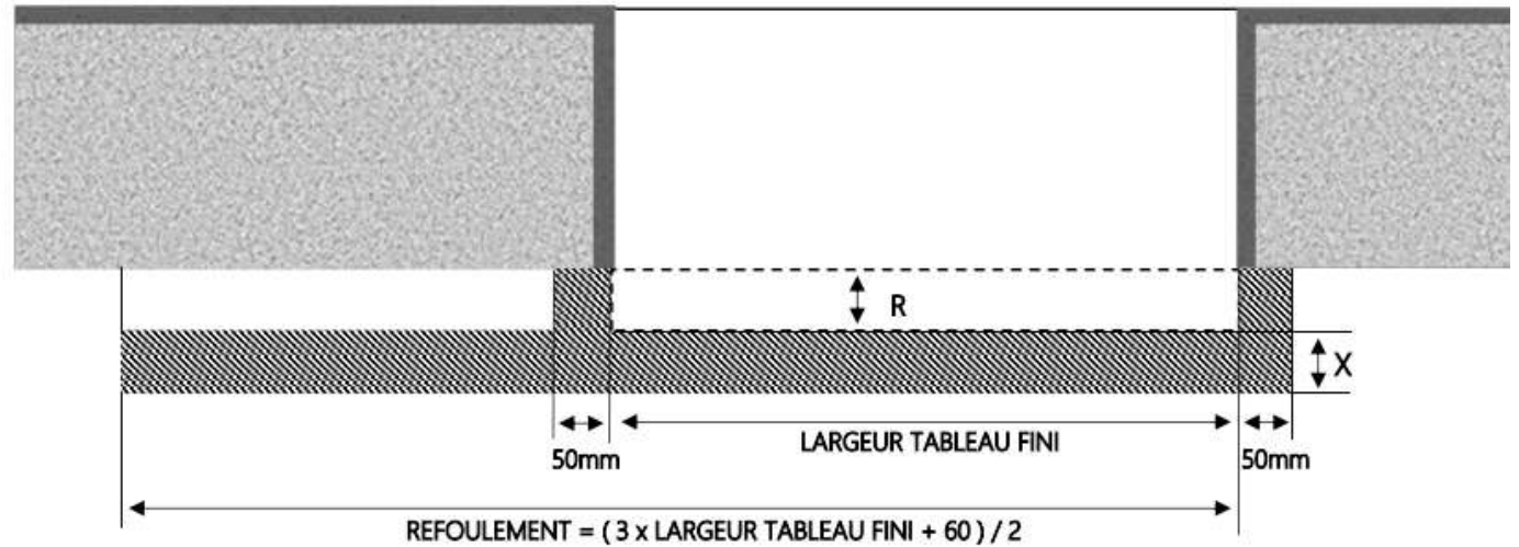
COUPE HORIZONTALE
