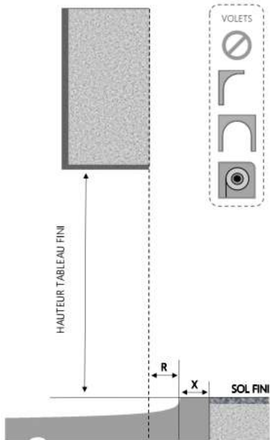
COUPE VERTICALE
