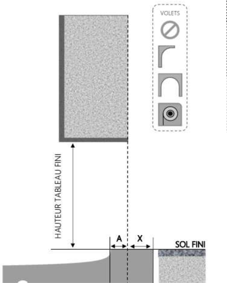
COUPE VERTICALE
