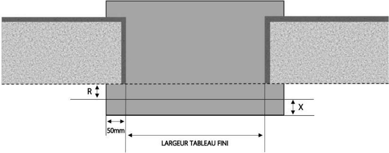
COUPE HORIZONTALE
