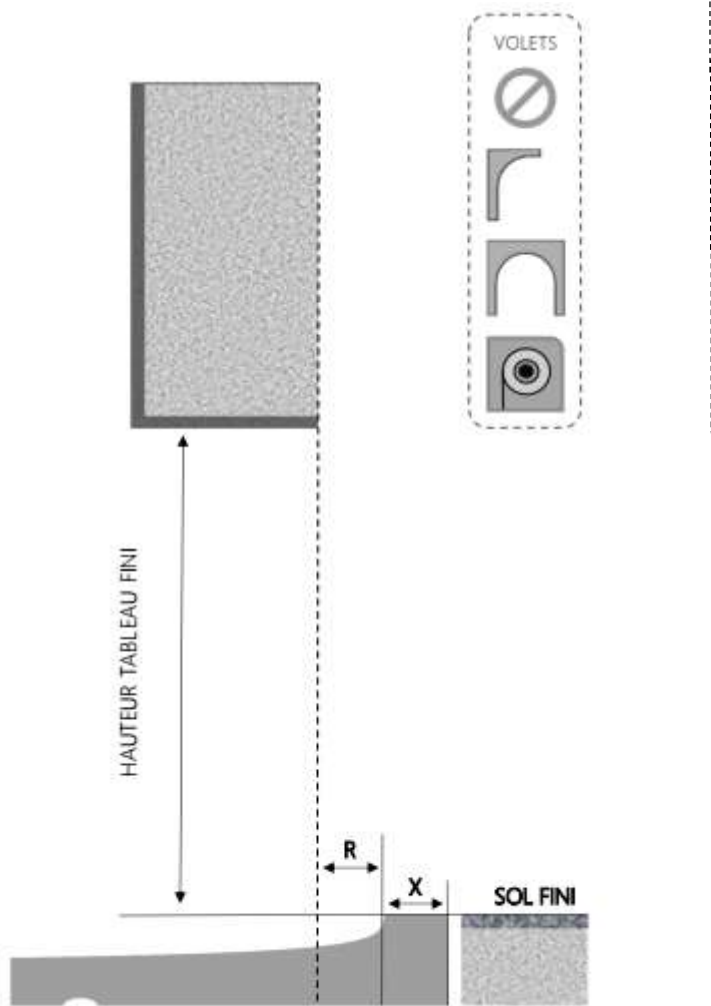
COUPE VERTICALE
