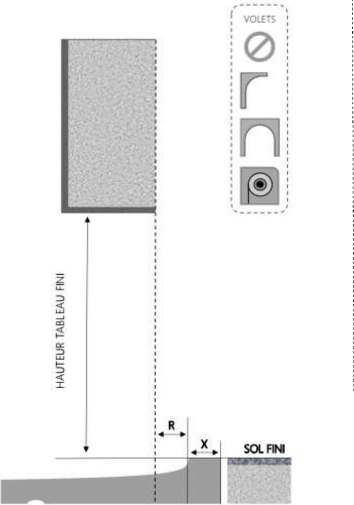
COUPE VERTICALE
