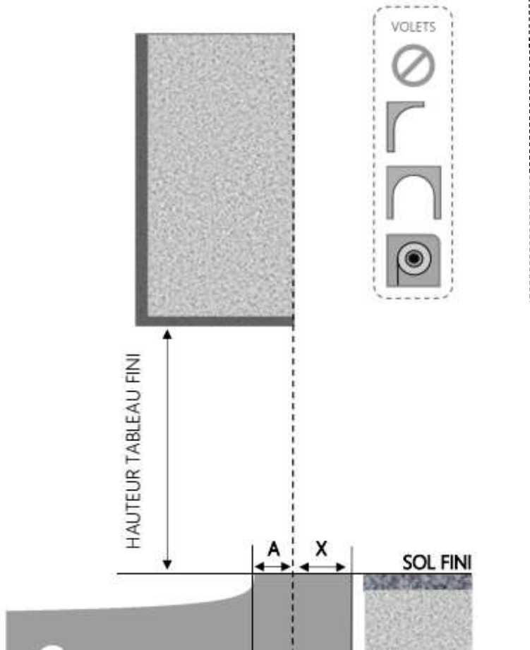
COUPE VERTICALE
