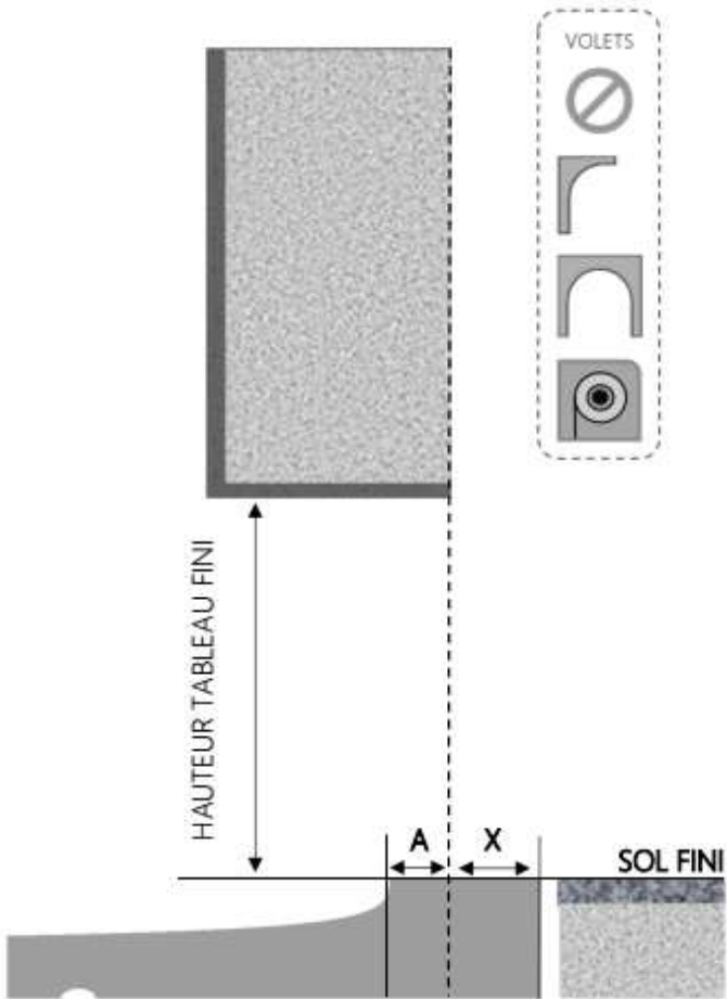
COUPE VERTICALE
