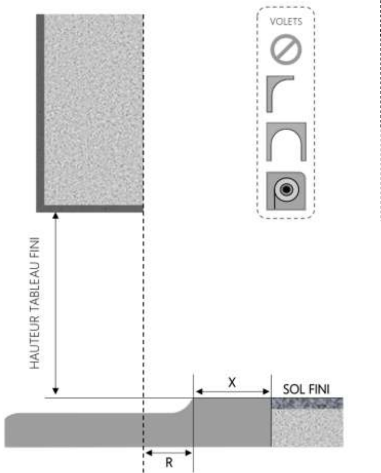
COUPE VERTICALE
