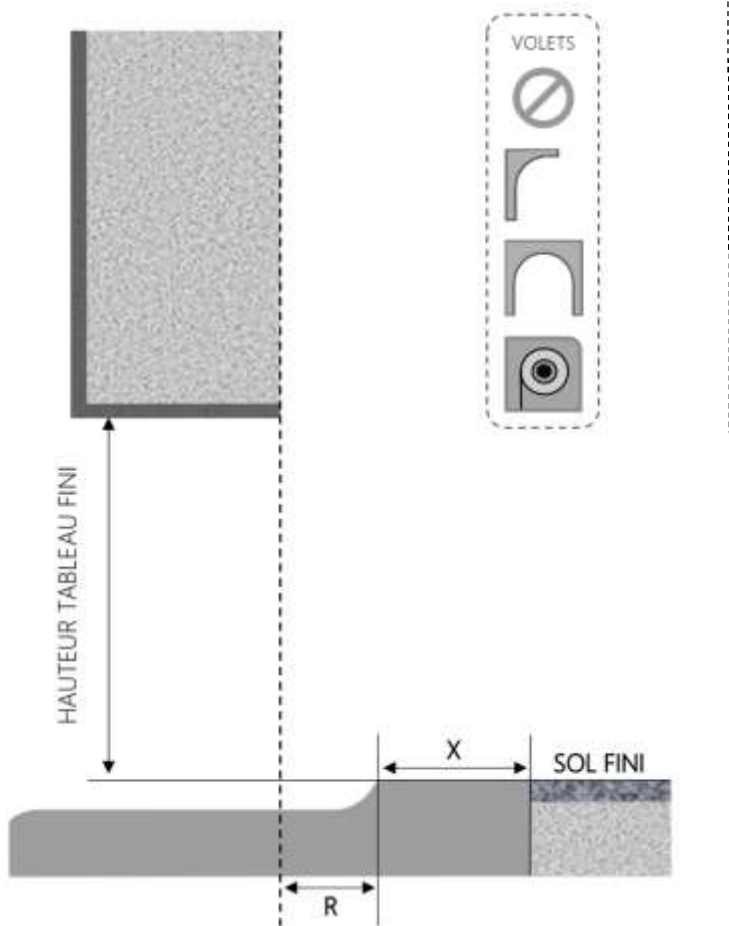
COUPE VERTICALE
