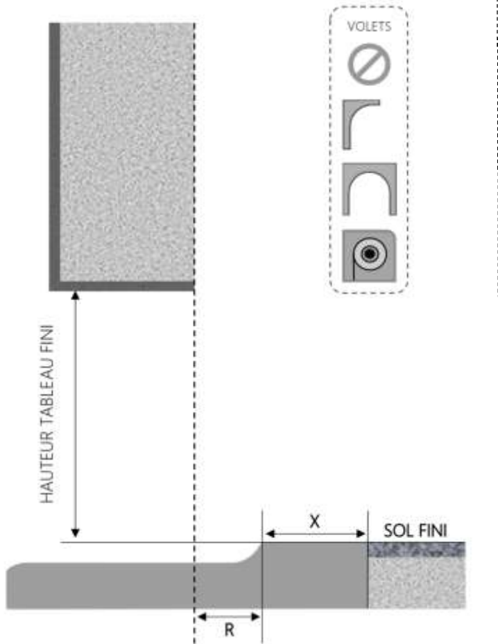
COUPE VERTICALE
