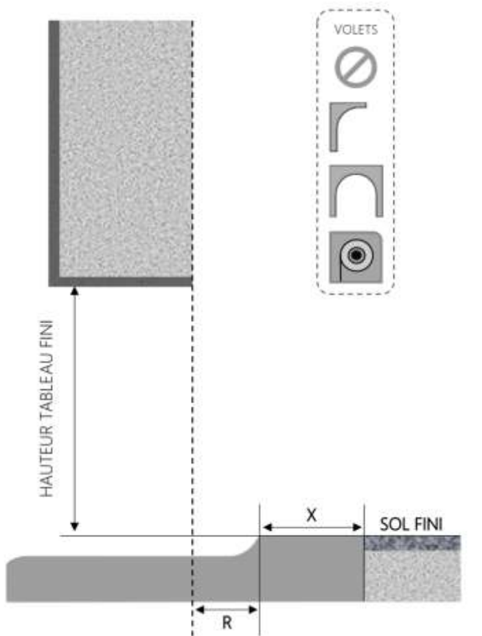
COUPE VERTICALE
