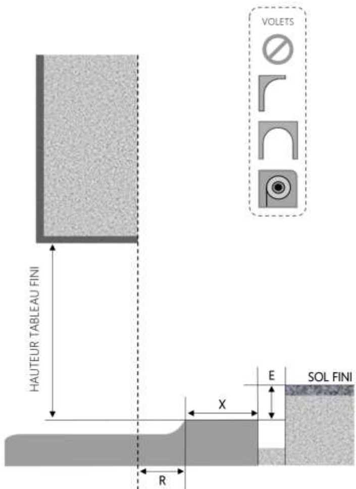
COUPE VERTICALE
