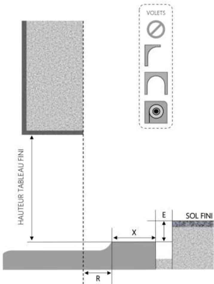
COUPE VERTICALE
