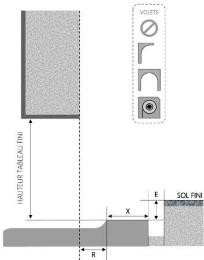
COUPE VERTICALE
