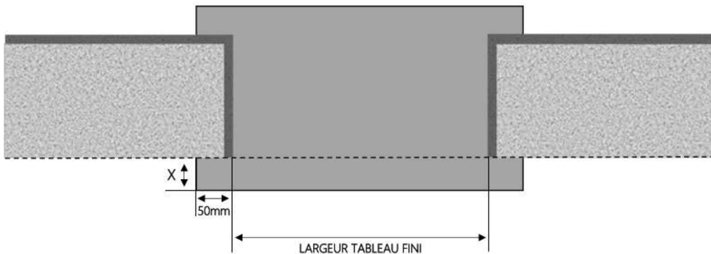
COUPE HORIZONTALE
