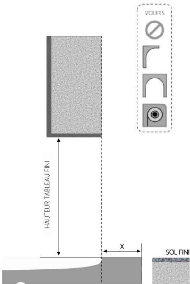
COUPE VERTICALE
