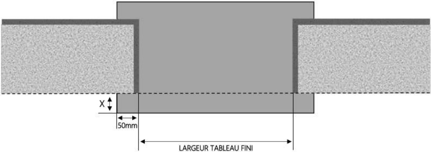
COUPE HORIZONTALE
