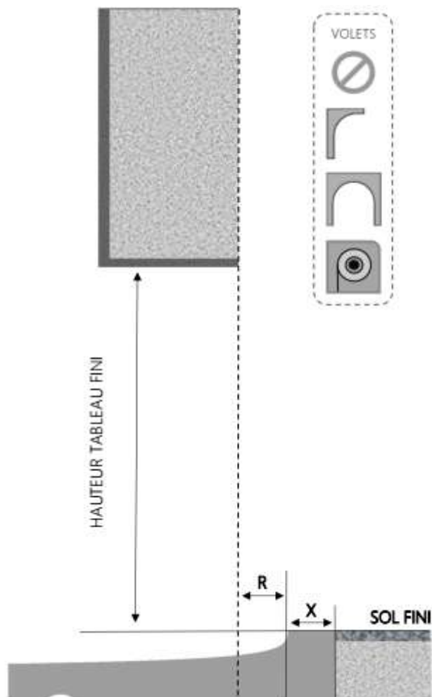
COUPE VERTICALE
