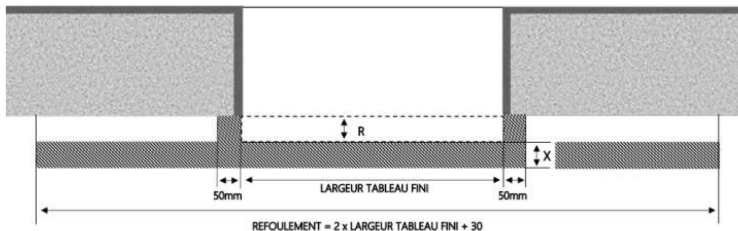
COUPE HORIZONTALE
